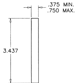
6 SIDE BAR
